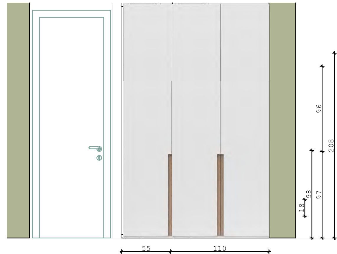
A-05 EXTERIOR ROPERO DORM. AUXILIAR 1:25
