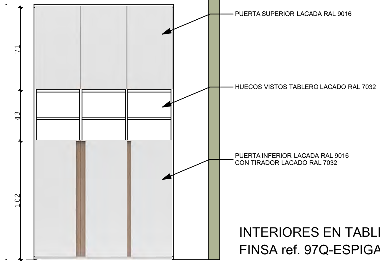
ALZADO EXTERIOR ARMARIO ZAPATERO
