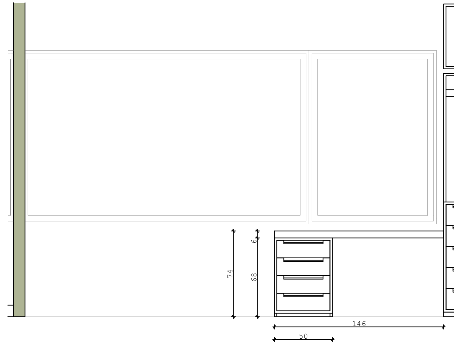
ALZADO ESCRITORIO DORMITORIO 2
