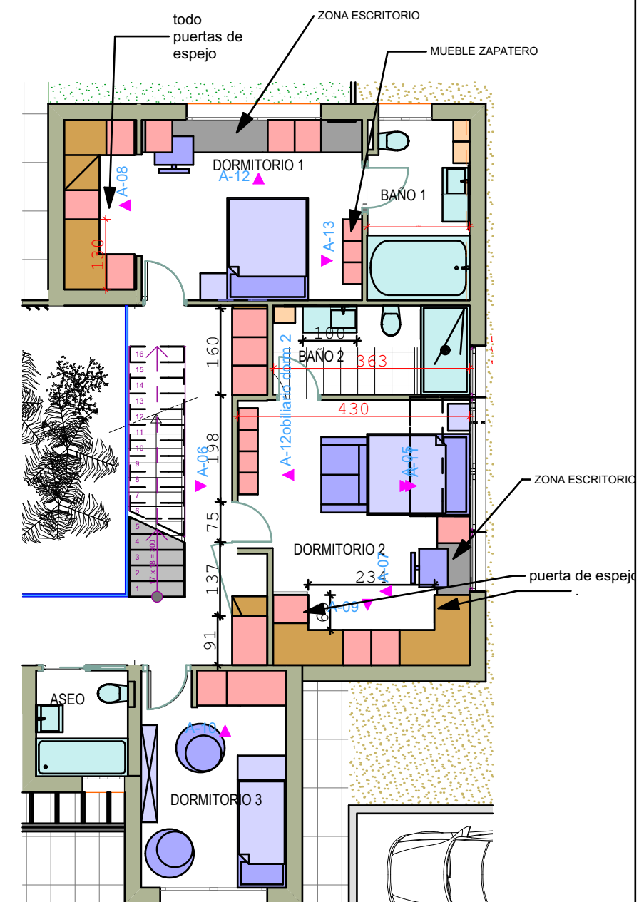
PLANTA BAJA ZONA DORMITORIOS 1:100
