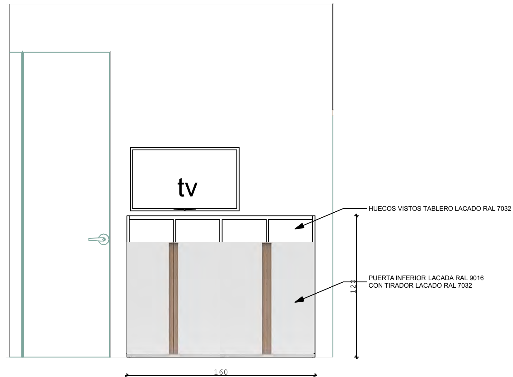
ALZADO EXTERIOR MUEBLE ZAPATERO
