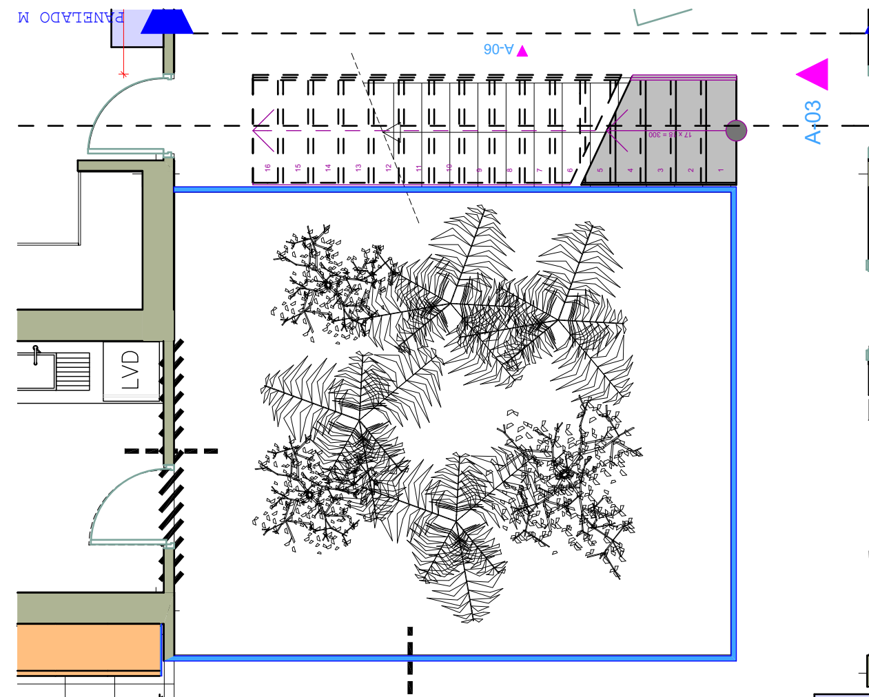
01.5 PLANTA ESCALERA 1:50
