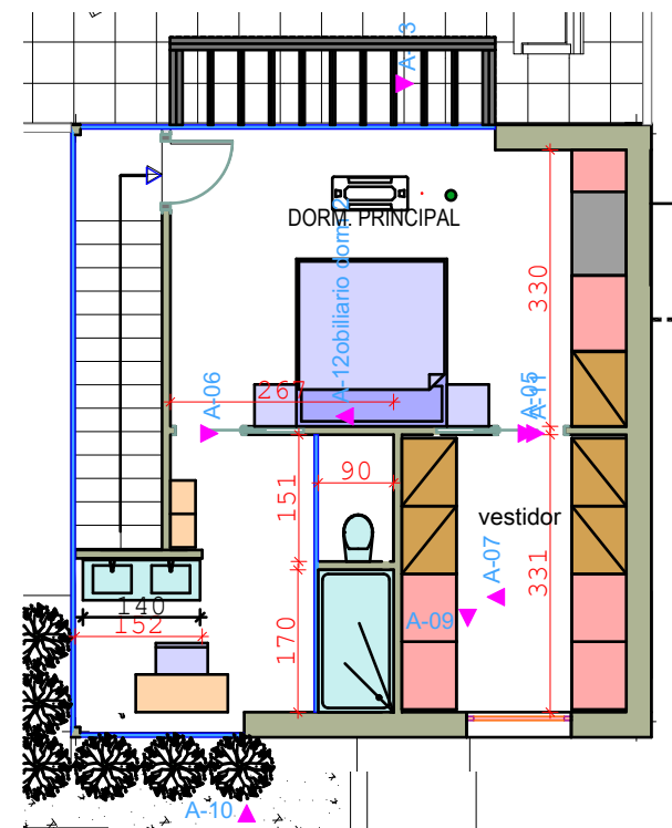
PLANTA DORMITORIO PRINCIPAL 1:100
