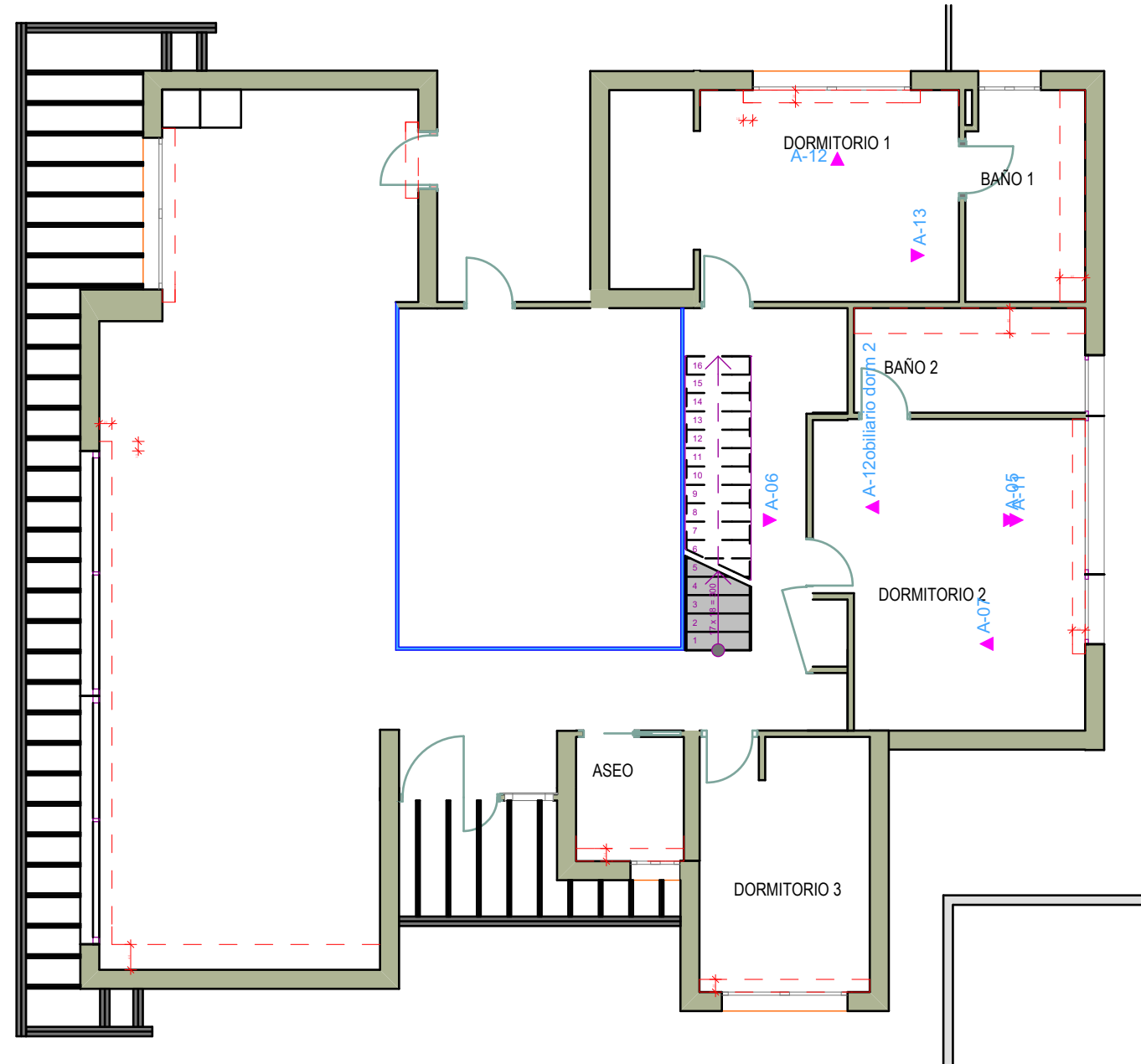
PLANO FOSEADOS PLANTA BAJA 01.10 1:100
