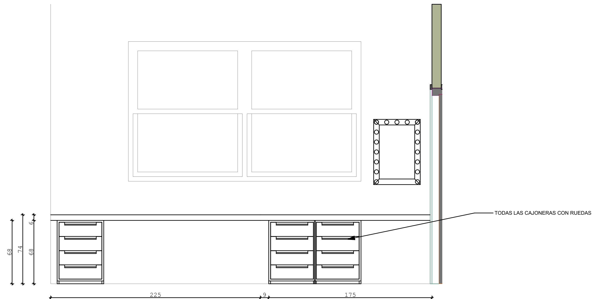
ALZADO ESCRITORIO DORMITORIO. 1
