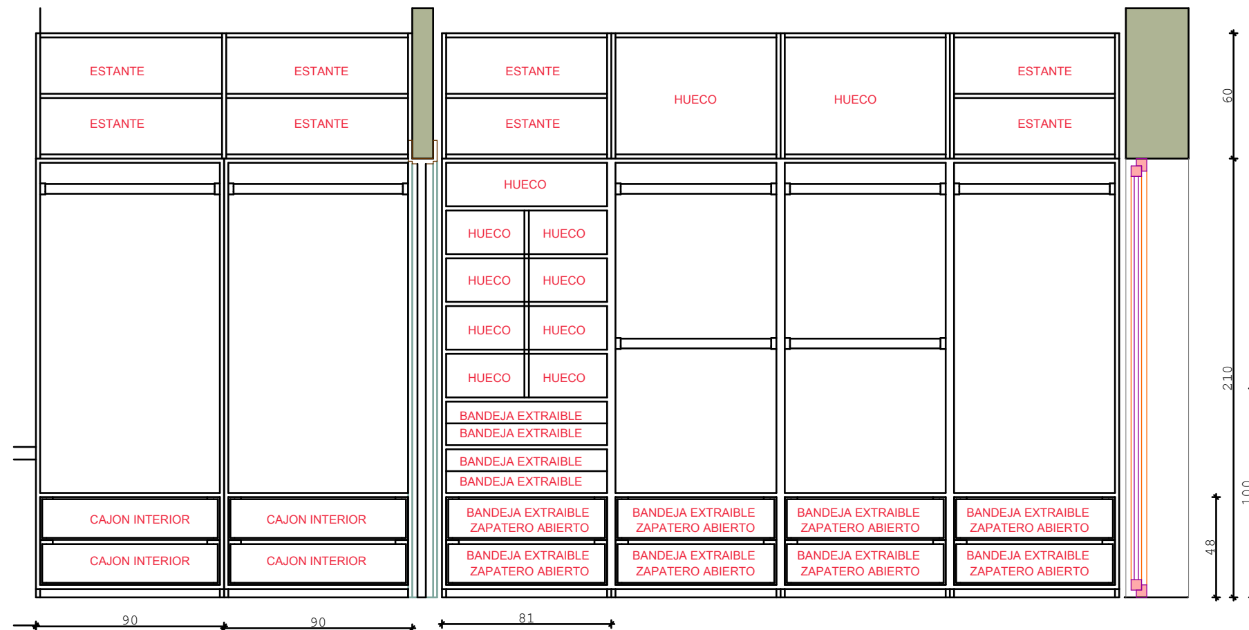
04.2 ALZADO ROPERO ALZADO EXTERIOR 1:25
