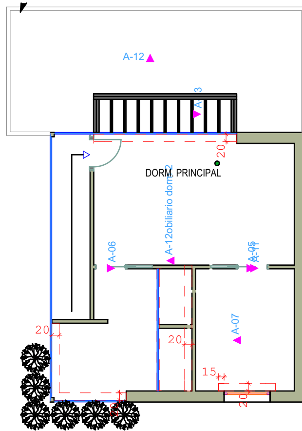
PLANO FOSEADOS PLANTA ALTA 01.10 1:100
