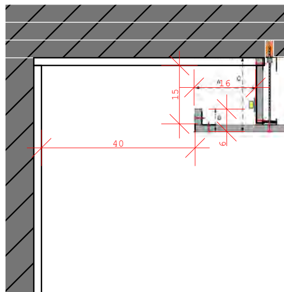
detalle foseado en baños 01.10 1:10
