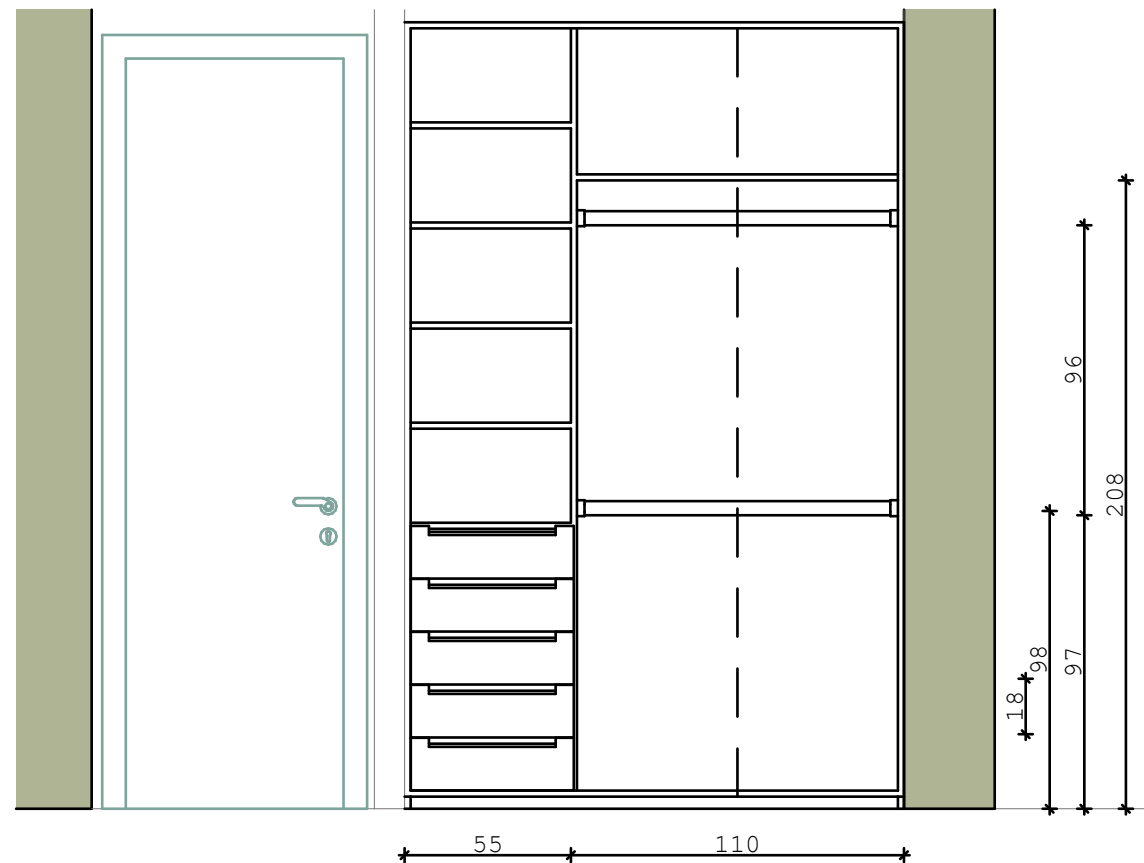
A-05 ALZADO INTERIORES ROPERO DORM. AUXILIAR 1:25
