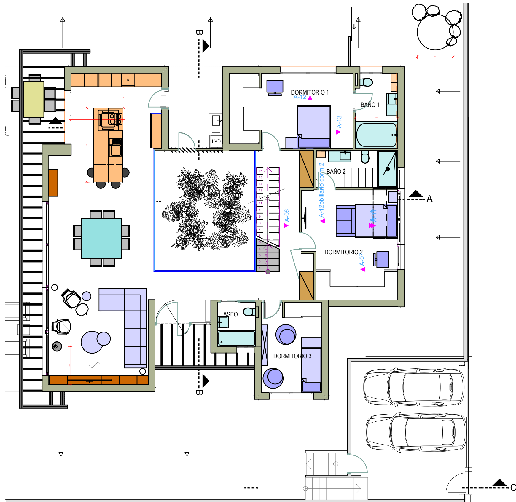
1 PLANTA BAJA DISTRIBUCIÓN
