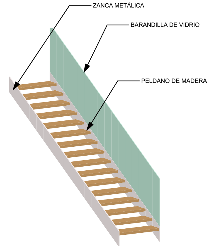
01.5 BOCETO ESCALERA 1:50
