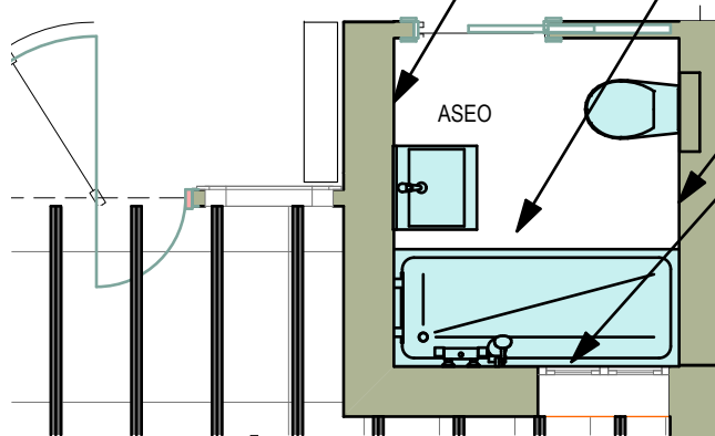
PLANTA ASEO
